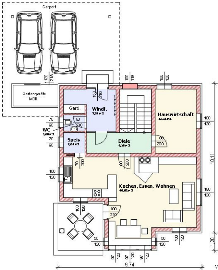
ERDGESCHOSS
