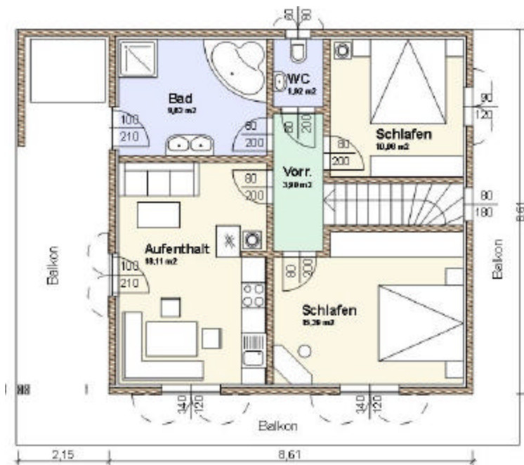
ERDGESCHOSS
