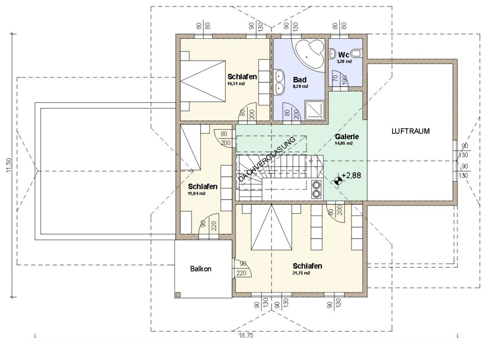
OBERGESCHOSS
